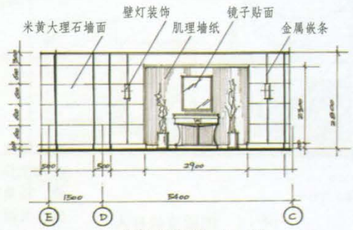
B向立面图 1:50
