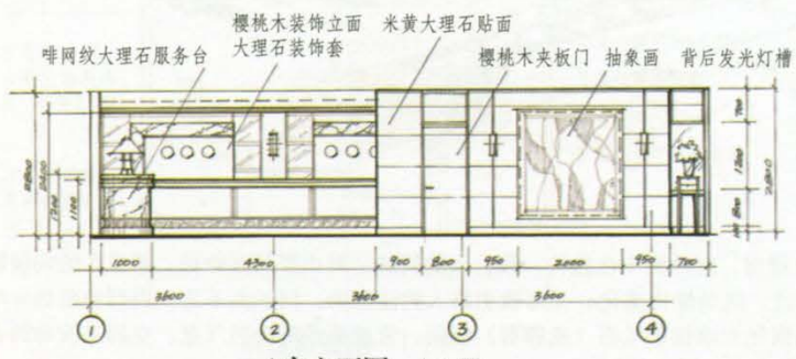
A向立面图 1:50
