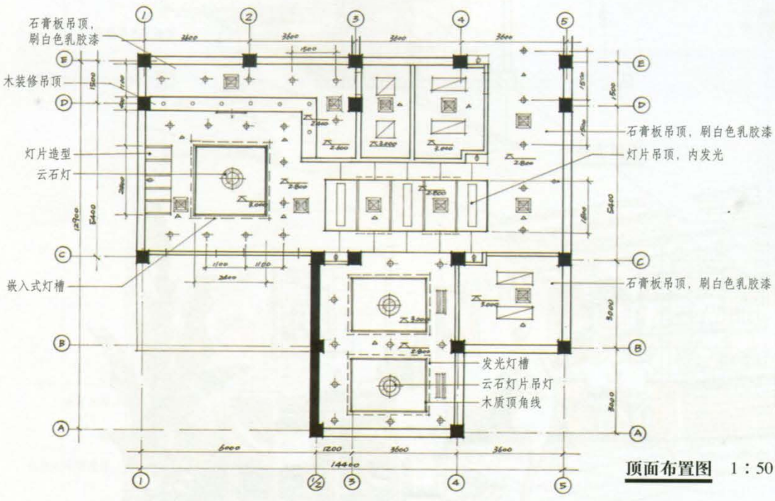
平面布置图 1:50
